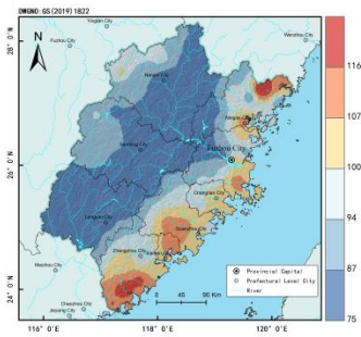
(d) 95th percentile rainfall
